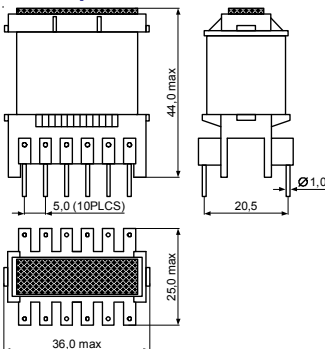
Серия SRV1105-XX
