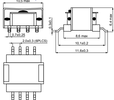
Серия SEV1934-XX
