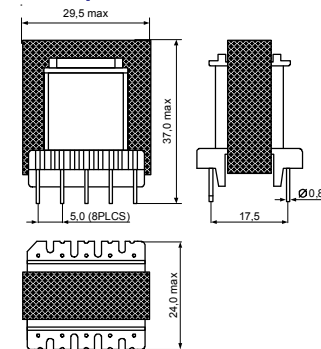
Серия SEV1601-XX
