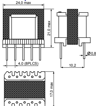
Серия SMV2201-XX
