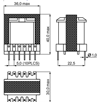
Серия SRV1103-XX
