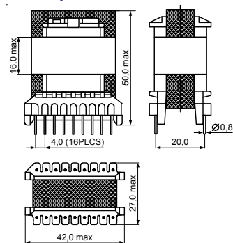
Серия SRV2812-XX
