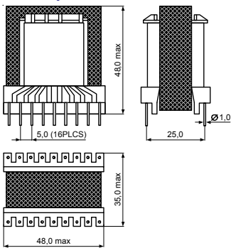
Серия SRV2905-XX
