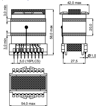
Серия SRV3404-XX
