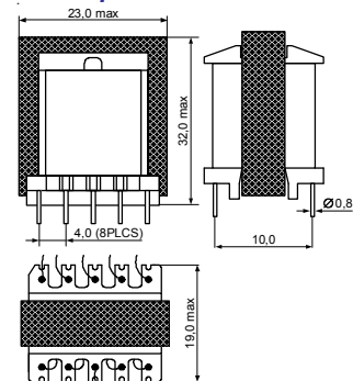
Серия SEV1934-XX
