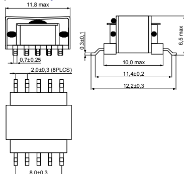
Серия SMV2201-XX
