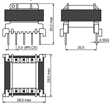
Серия SEH2516-XX
